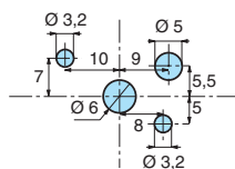
Fissaggio dal retro
