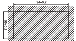
Foratura pannello con uso della mascherina A70R Cut out with use of A70R frame
