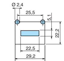
Fissaggio dal retro
