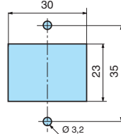
Fissaggio dal retro Rear fixing
